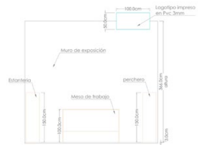
ALZADO
